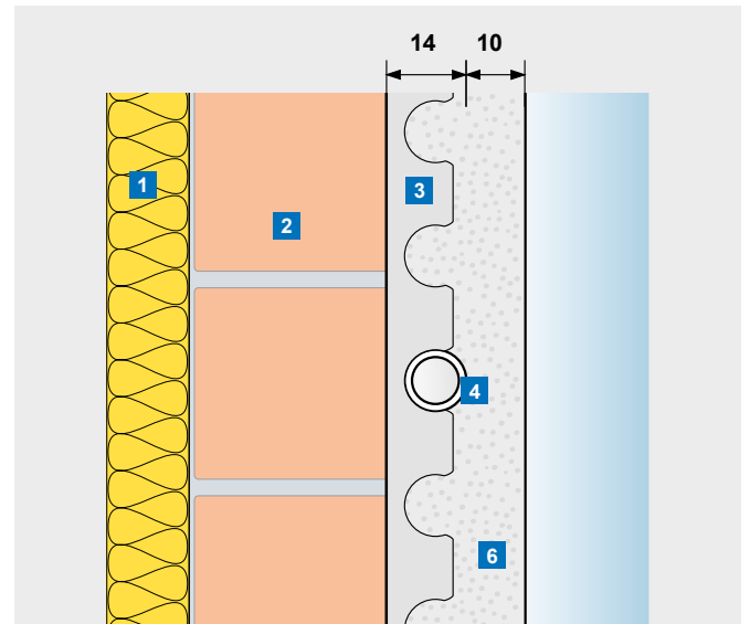
Shematski prikaz Uponsorovog Fix sustava na zidu
