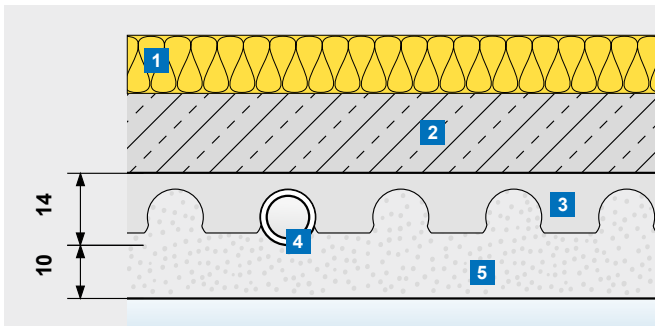
Shematski prikaz Uponsorovog Fix sistema na stropu
